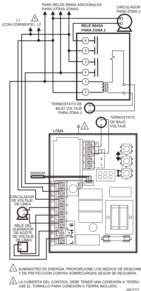
Fig. 10. Sistema de zonas múltiples del L7224U con conexiones para circuladores.
