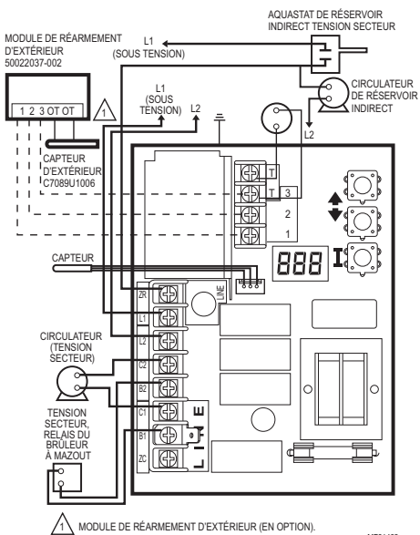
Fig. 9. Système à zone de chauffage unique avec circulateurs et réservoir d'eau indirect L7224U. Module de réarmement d'extérieur facultatif.
