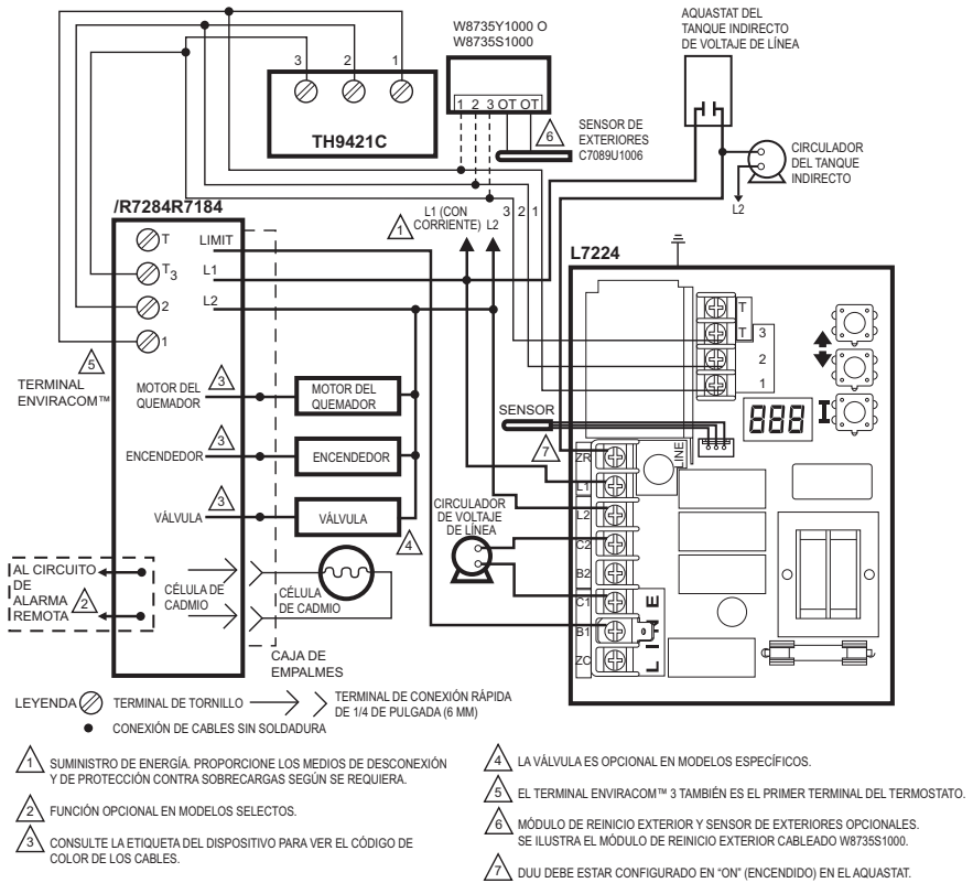
Fig. 12. L7224U con sistema de una zona con circulador, tanque de agua indirecta y termostato EnviraCOM™.
