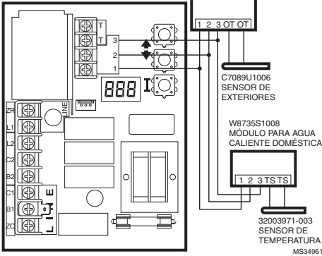
Fig. 6. Cableado del módulo de reinicio exterior y del módulo para agua caliente doméstica.
